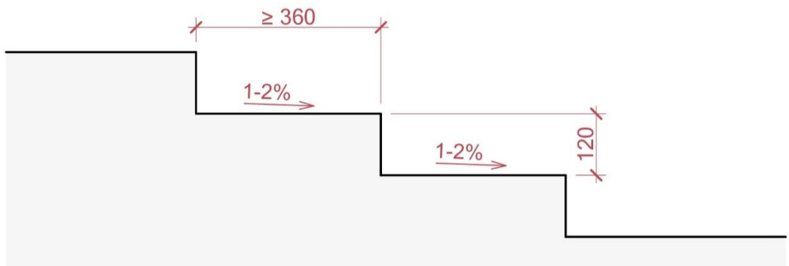
Рисунок 46 - Параметри відкритих сходів та ґанків
