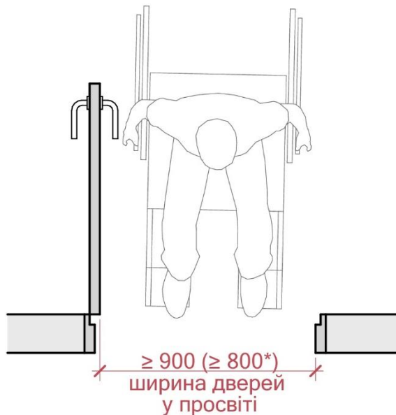
Рисунок 7г – Ширина дверей у просвіті
