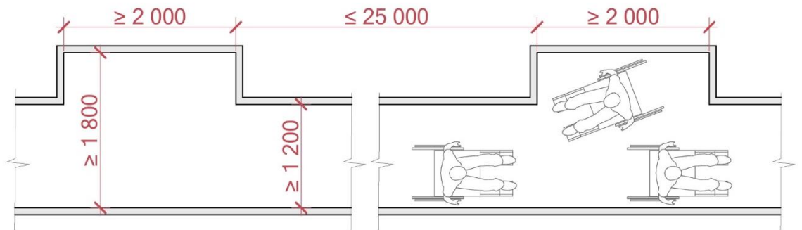
Рисунок 1в - Приклад влаштування пішохідної доріжки з роз'їзними кишенями
