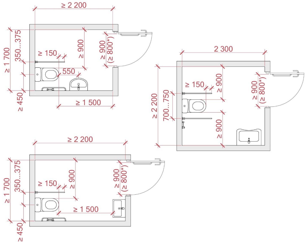
Рисунок 41в — Приклади проектних рішень універсального санітарно-гігієнічного
