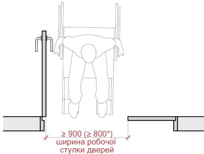
Рисунок 7е – Ширина робочої частини (стулки) в простві
